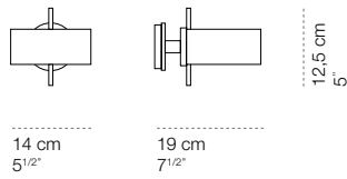
newComponi200 uno parete
