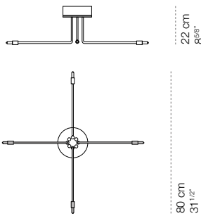
CiniLightSystem composizione 4C
