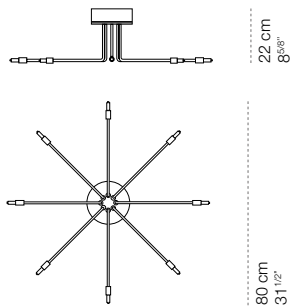
CiniLightSystem composizione 8C
