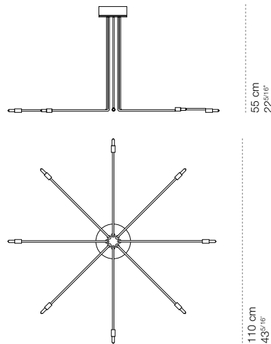
CiniLightSystem composizione 8L
